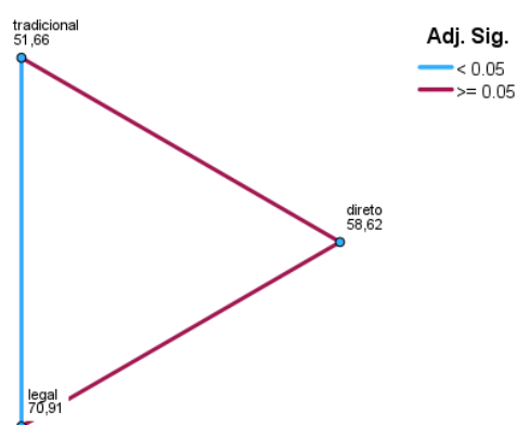
Gráfico 6 – Teste pairwise
